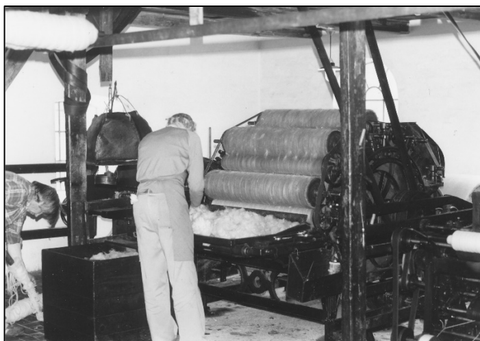
Kartemaskine på Rebstrup Uldspinderi, her opstillet i Raadvad
